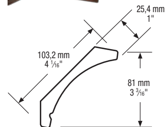
9447 Ogee Longueur / Length: 9 pi/ft
