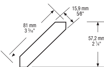
9446 Ogee Longueur / Length: 9 pi/ft
