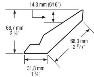
9443 Moulure de Tête / Crown moulding Longueur / Length: 9 pi/ft
